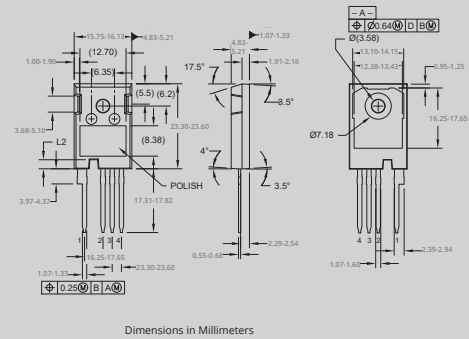
TO-247-4L Notch
