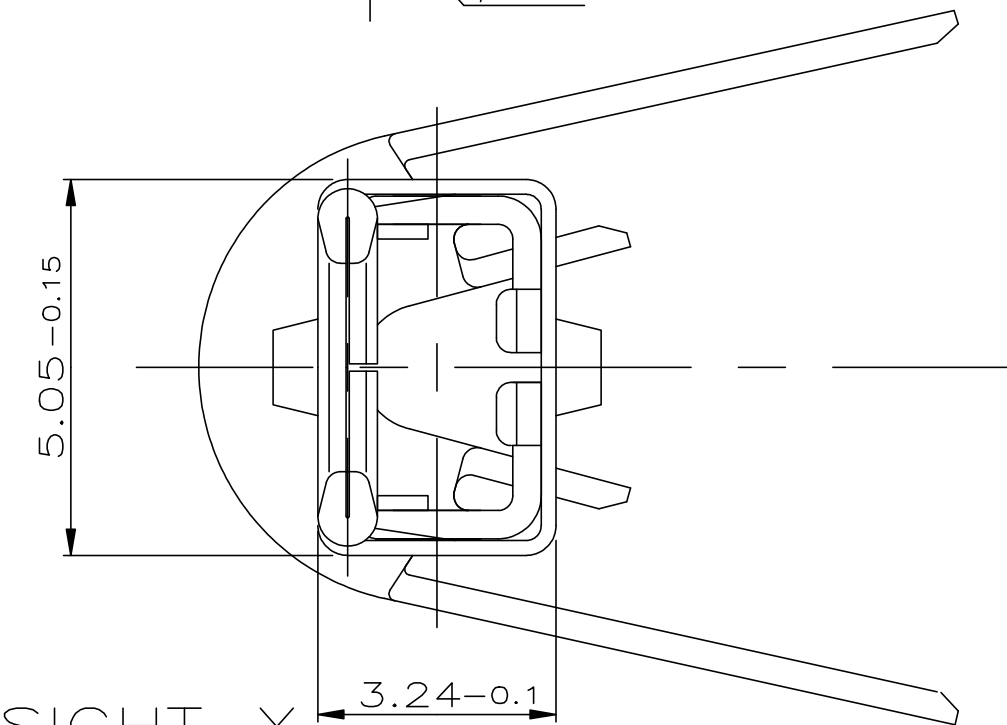
ANSICHT X
