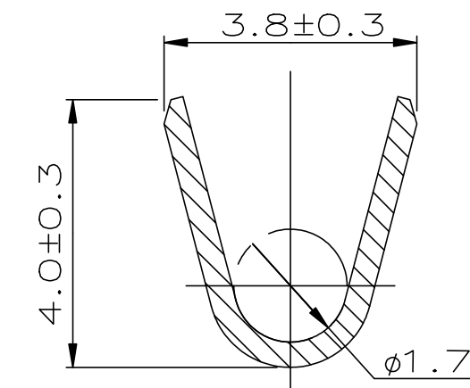
Schnitt C-C
