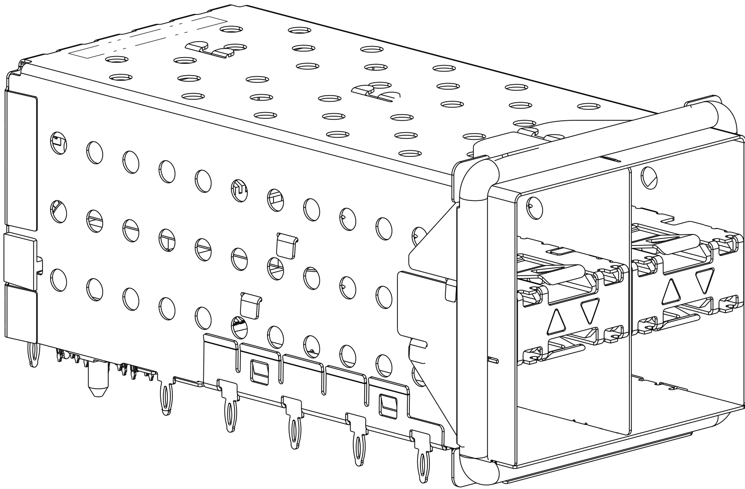
2007417-6 AND 1-2007417-6 SCALE 3:1
