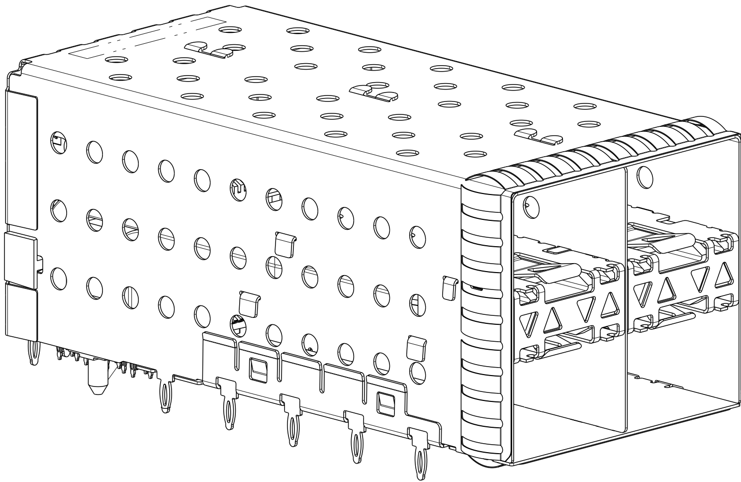
2007637-5, 1-2007637-5, 3-2007637-5 SCALE 3:1
