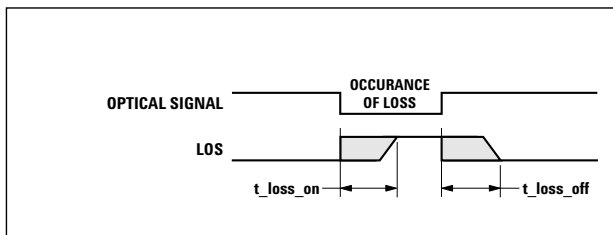
t_{\text{loss-on}} & t_{\text{loss-off}}
