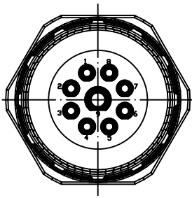
9-Pole (8+1)
