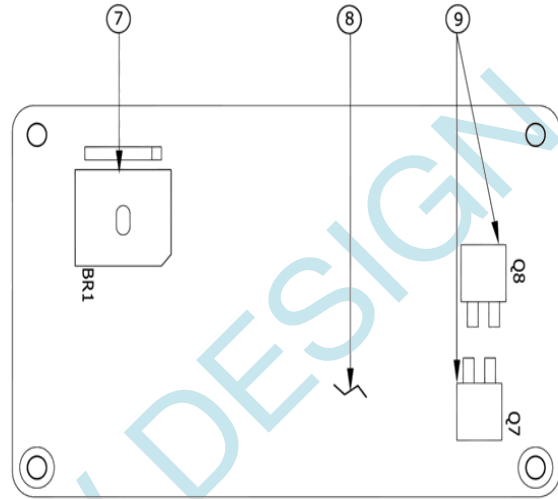
BOTTOM PCB
