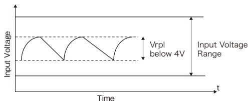
Fig.1-1 Input Ripple Voltage
